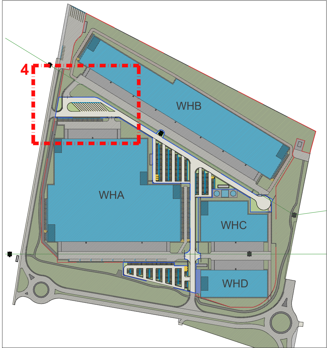
Keyplan - AIU 1 1 : 4.000
