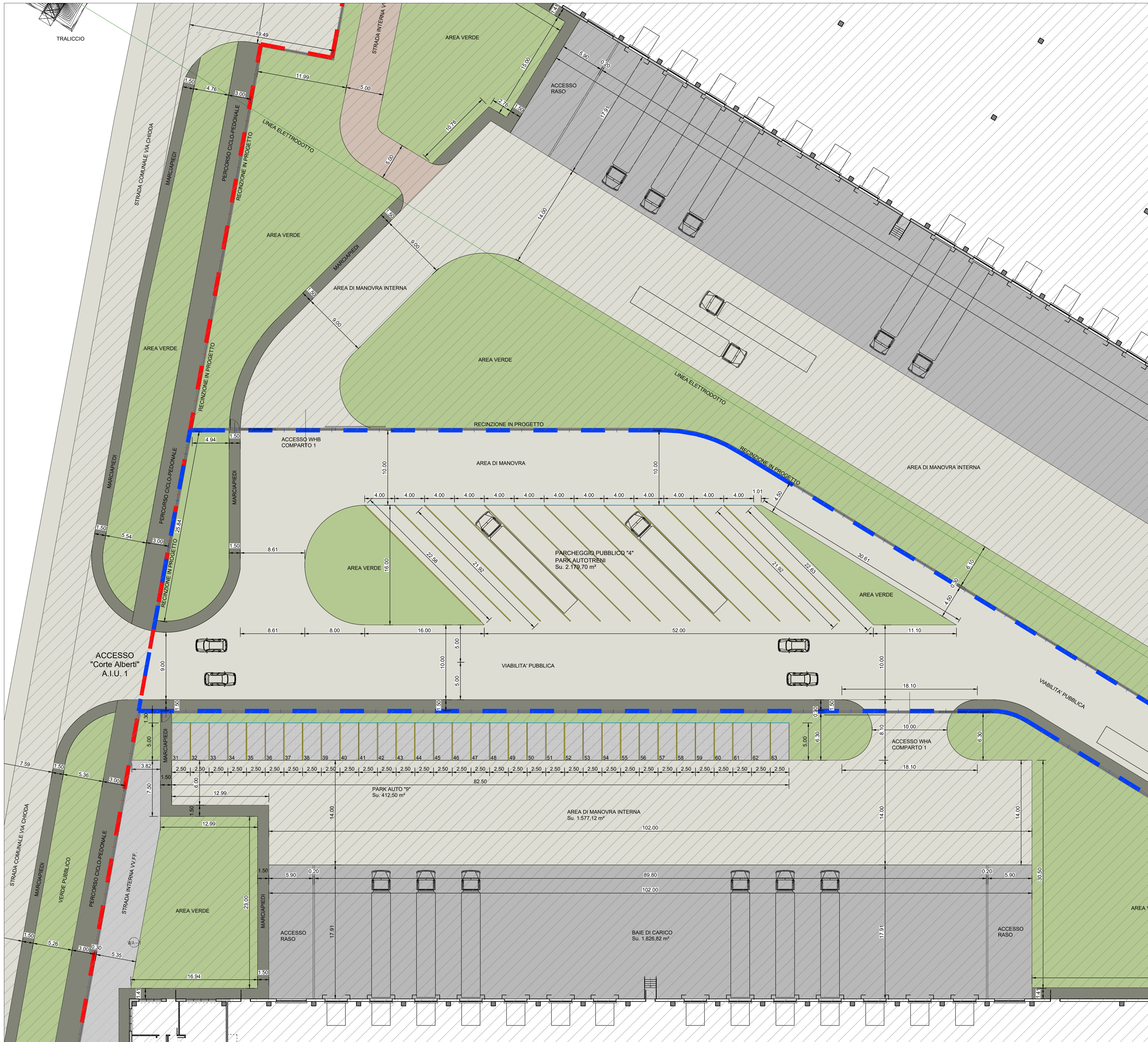
INGRANDIMENTO AREE ESTERNE 04 Scala 1 : 250
